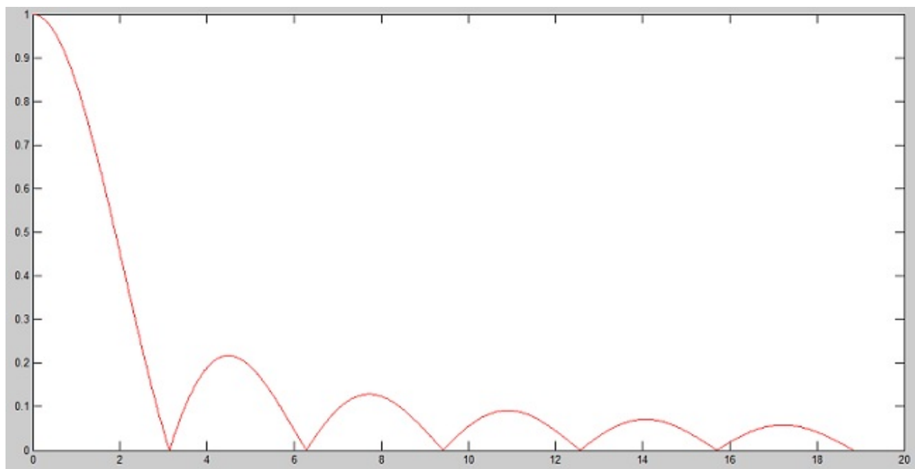
Représentation graphique de la fonction y = \text{abs}(\sin(x))/x
