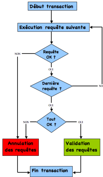
FIGURE 28.1 – Schéma d’une transaction
