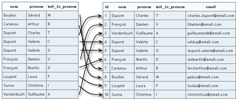
FIGURE 11.3 – Index sur trois colonnes
