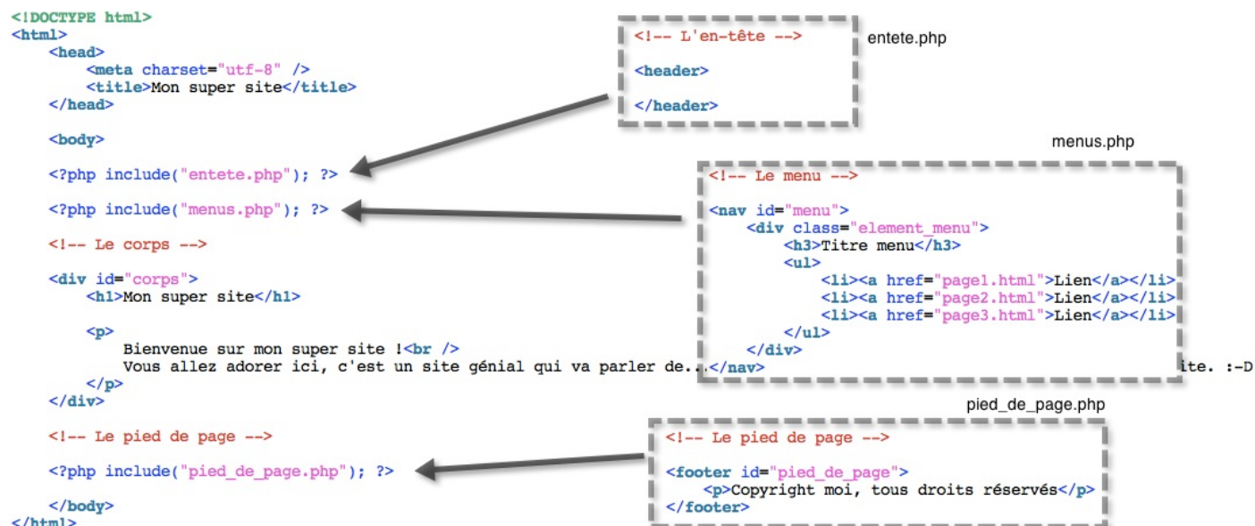
Les includes en pratique
