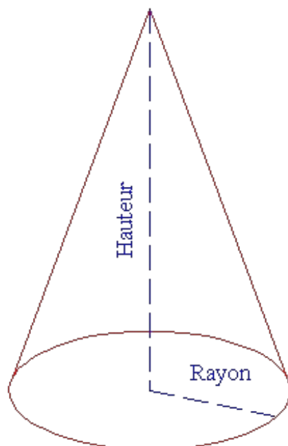
Représentation d'un cône
