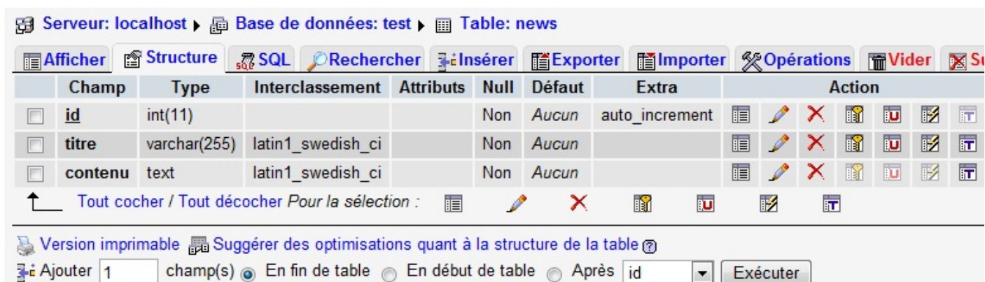
Structure de la table news
